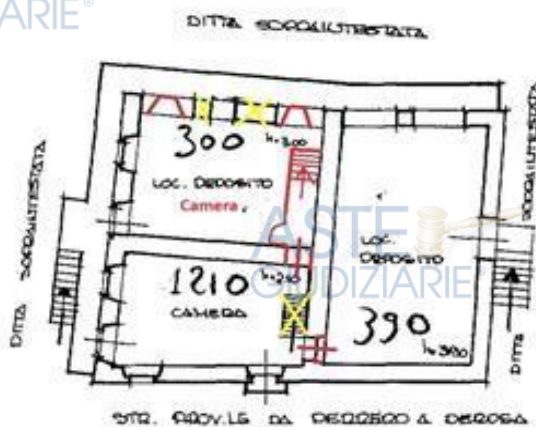
PIANO PRIMO ORIENTAMENTO
