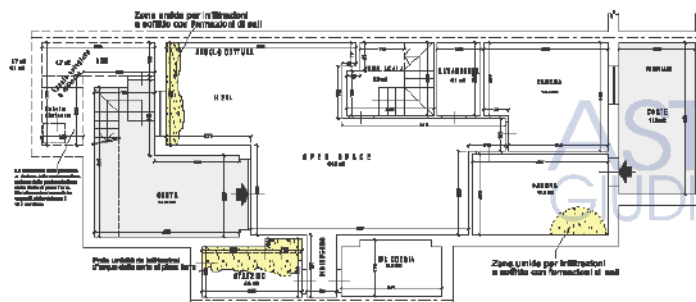
PIANTA PIANO SOTTOSTRADA SUP. LORDA 102,6 mq (comprese le scale e il locale autocarino)
