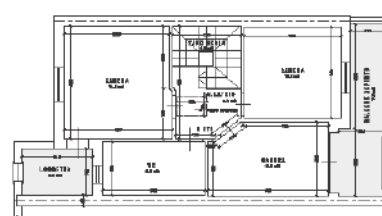
PIANTA PIANO PRIMO SUP. L.ORDA 212 m 2 (compresi i balconi)
