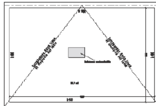
PIANTA DEL SOTTOTETTO SUP. LORDA 68,4 mq
