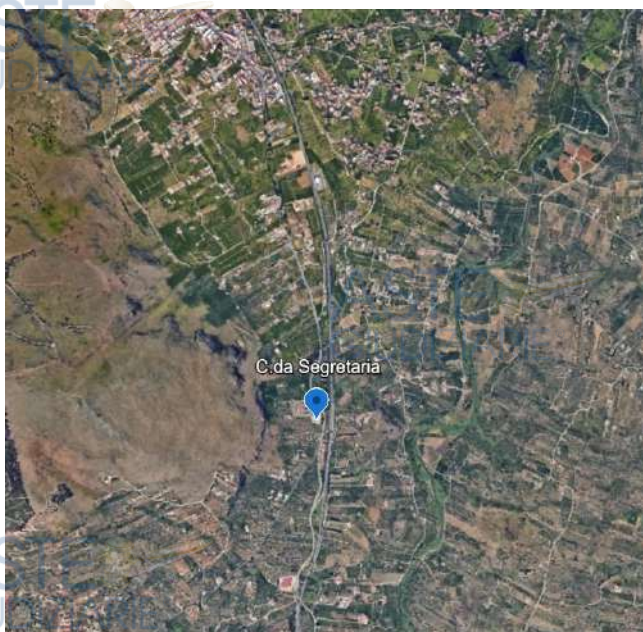
FIGURA 2 – STRALCIO SATELLITARE
