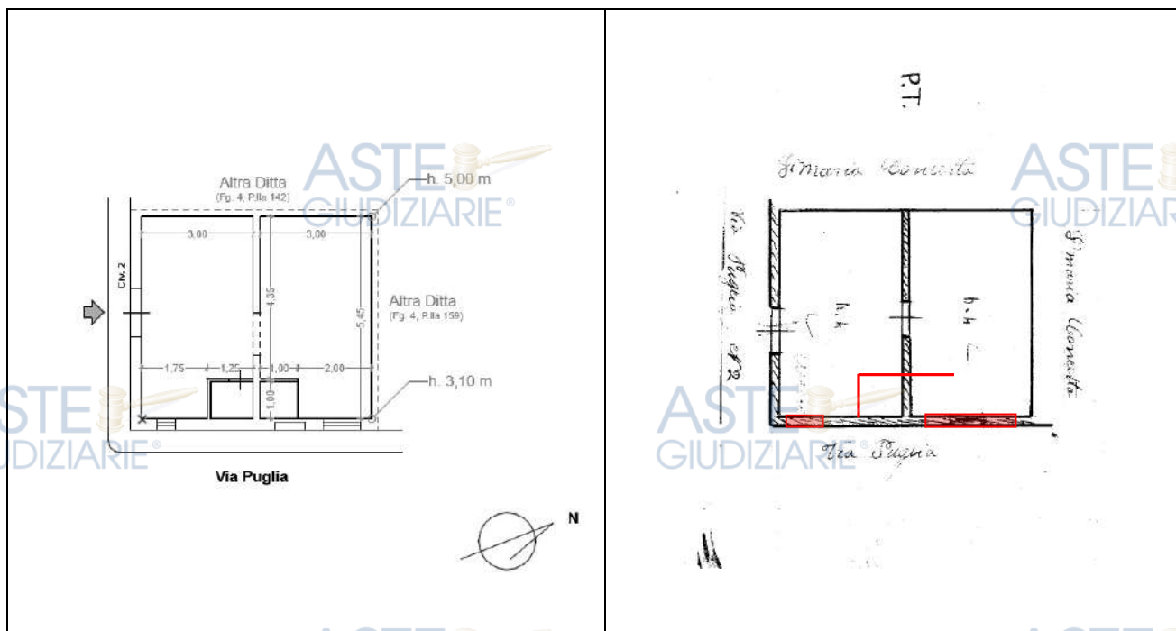
FIGURA 8- PLANIMETRIA DI CONFRONTO RILIEVO DELLO STATO DI FATTO E PLANIMETRIA CATASTALE
