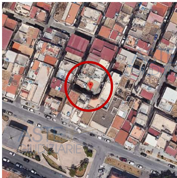
FIGURA 1 – STRALCIO SATELLITARE
