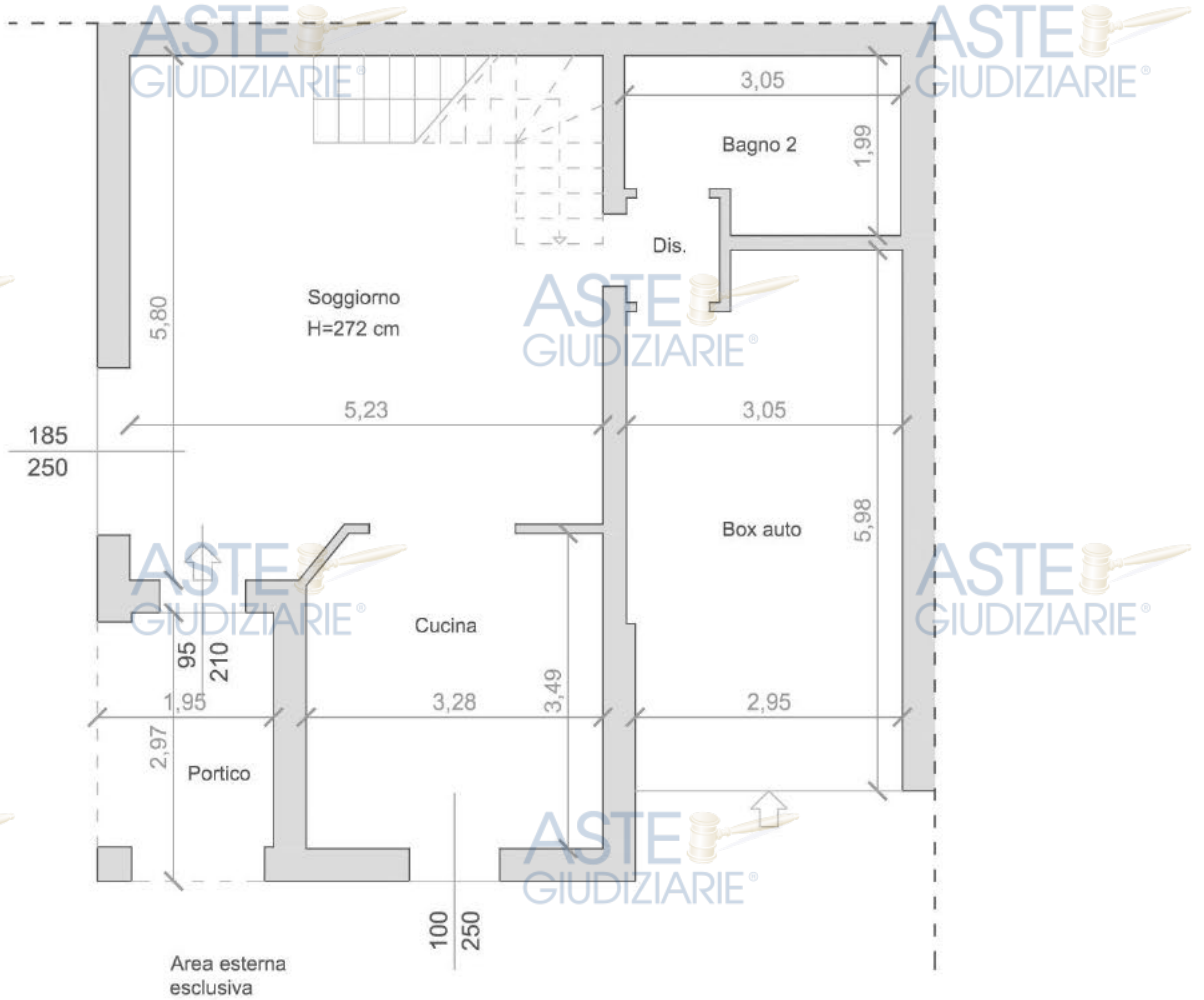
Fot. 1 - Pianta Piano terra
