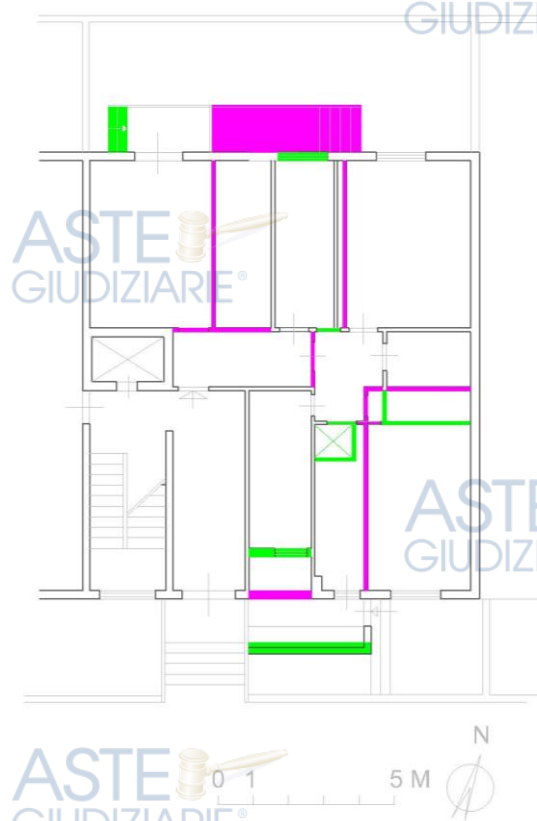
Planimetria di rilievo attuale con indicazione delle difformità rispetto al grafico di progetto autorizzato e alla planimetria catastale
