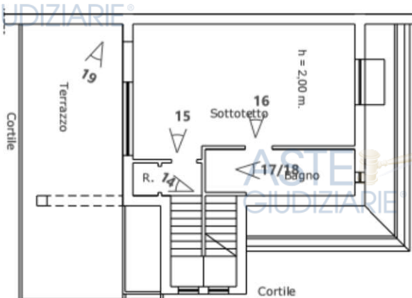
PLANIMETRIA PIANO SECONDO (SOTTOTETTO)
