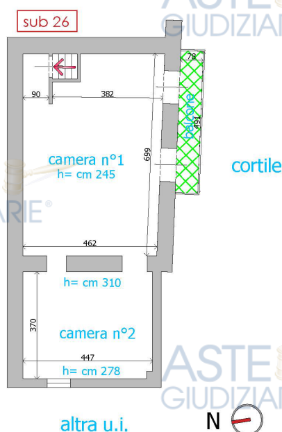
Planimetria dell'immobile pignorato SUB 26 (piano secondo)
