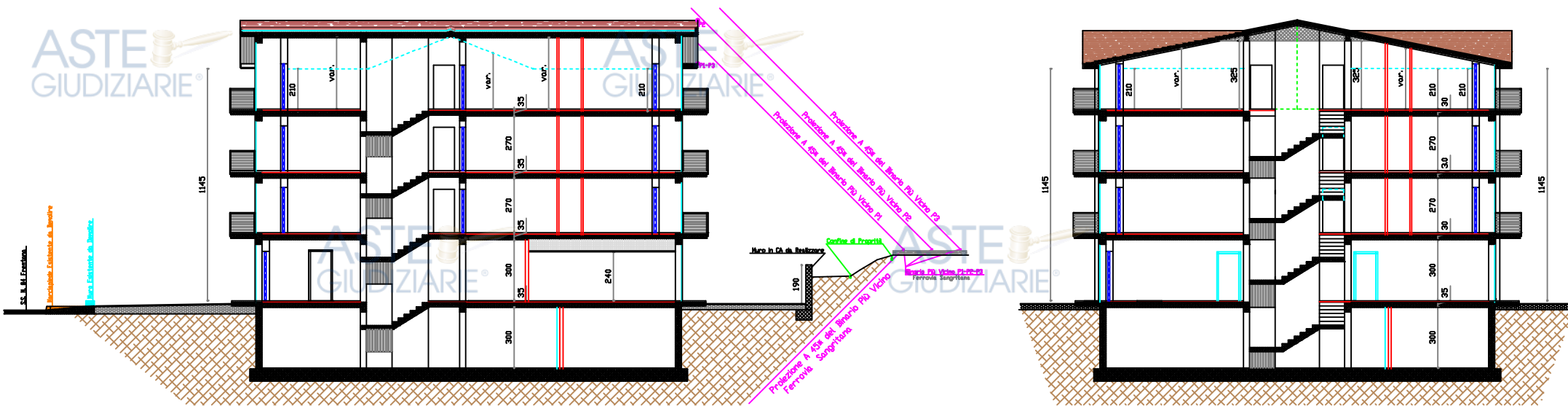
Sezione X-X
