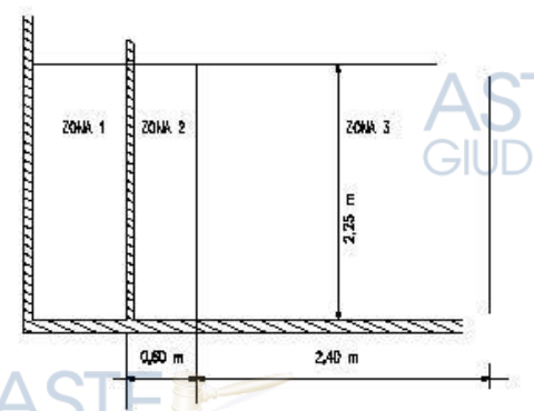
DOCCIA SENZA PIATTO, MA CON PARETE FISSA
