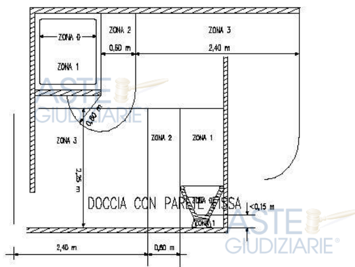
VARIANTE CON VANO SOTTOVASCA
