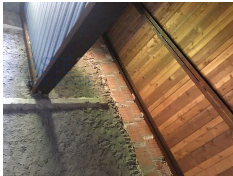
Particolare solai in legno e ferro
