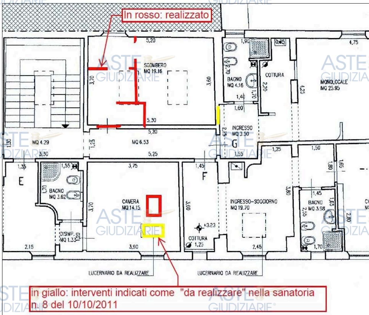
Fig. 2 – porzione di pianta p. primo (non in scala) con indicazione qualitativa delle difformità osservate
