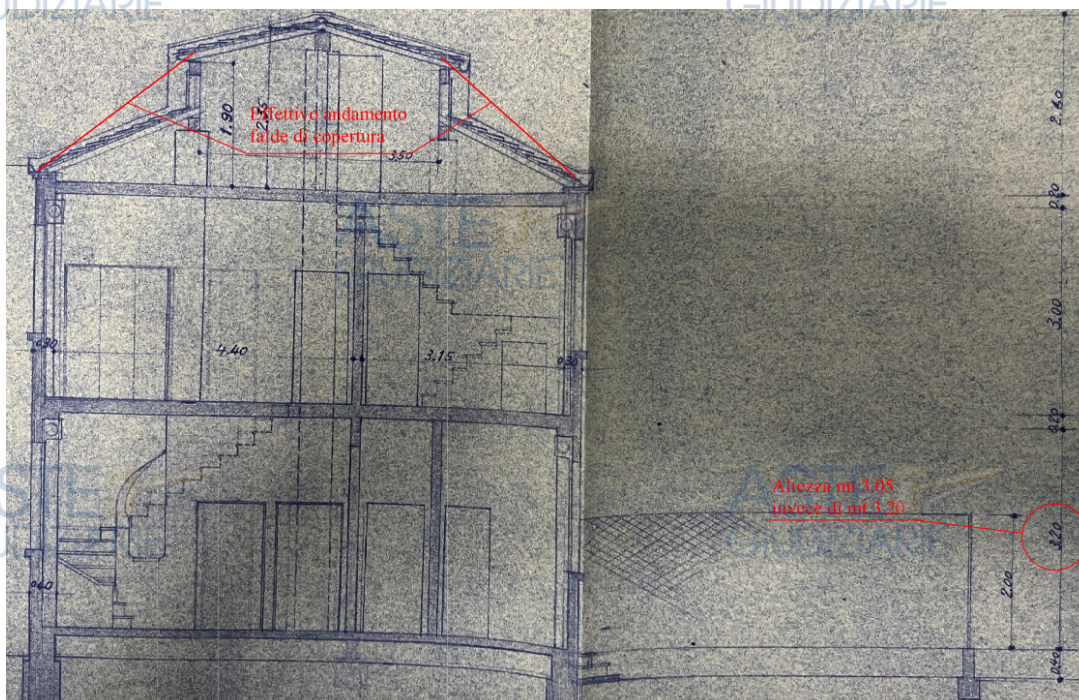
Sezione
