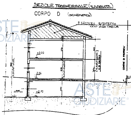
Estratto progetto - sezione tipo
