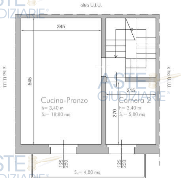
Via Mario Rapisardi Pianta piano primo
