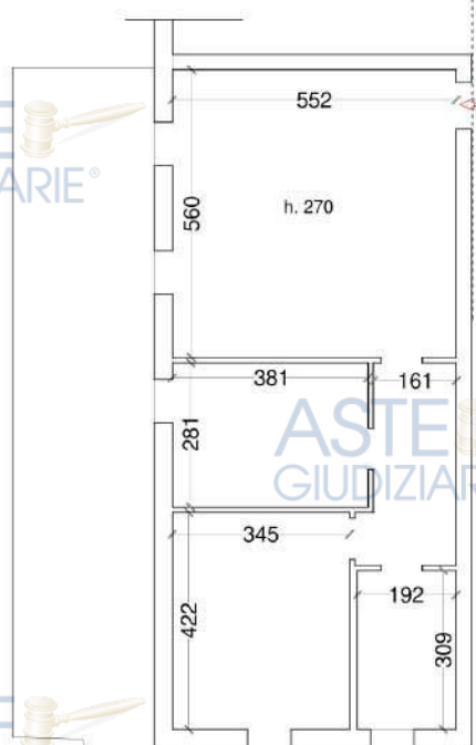
RILIEVO APPARTAMENTO SUB 2 P. TERRA
