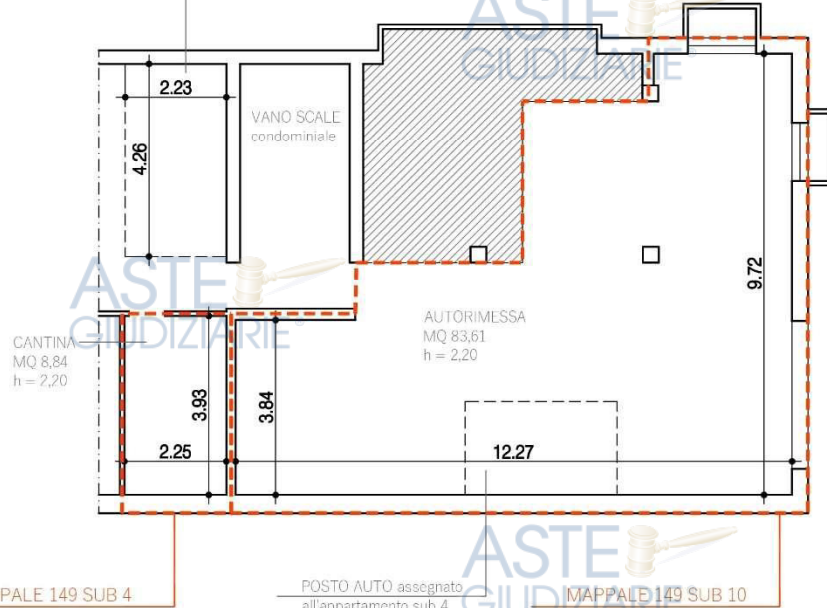
FOGLIO 108, PARTICELLA 149 SUB 4 E SUB 10 - PIANO INTERRATO
