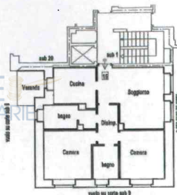
Pianta Piano quarto - h 2.70
