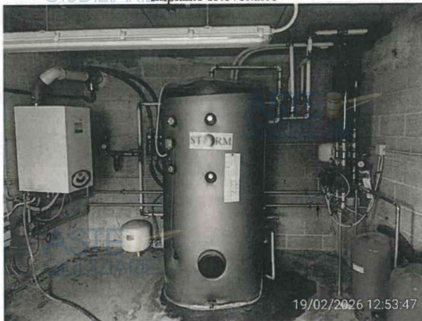
Centrale termica
