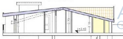
STRALCIO SEZIONE A-A DI PROGETTO
