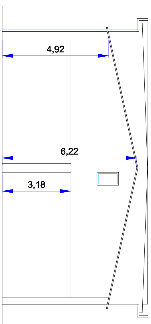
sezione A-A
