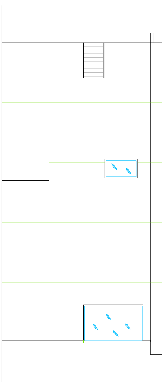
prospetto ovest
