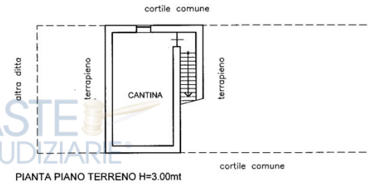
PIANTA PIANO TERRENO H=3.00mt
