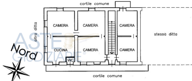
PIANTA PIANO TERRENO H=3.00mt
