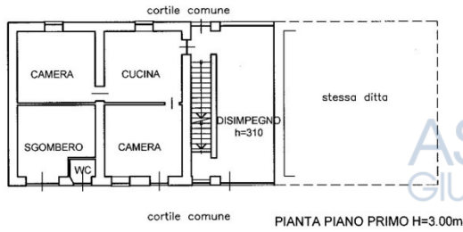
PIANTA PIANO PRIMO H=3.00mt
