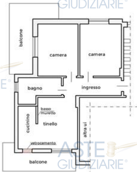
Rilievo qualitativo dell'u.i. a cura della scrivente, indicativo dello stato dei luoghi al momento del sopralluogo
