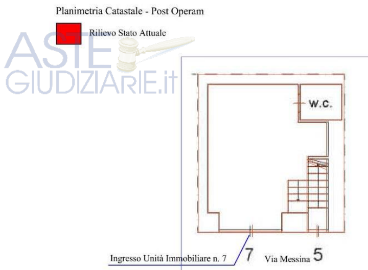
Rilievo Stato di fatto - Planimetria Catastale Piano Terra - Post Operam
