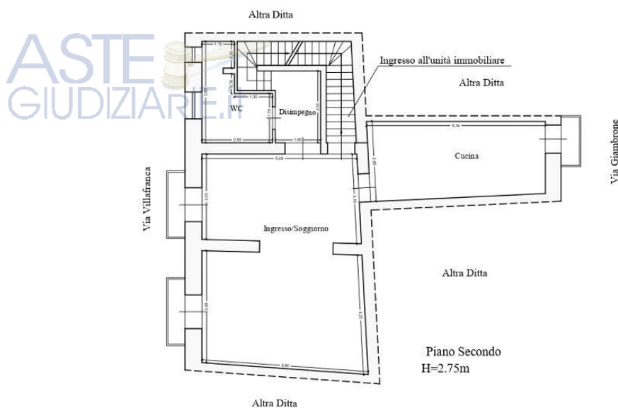
Rilievo Stato di fatto Piano Secondo
