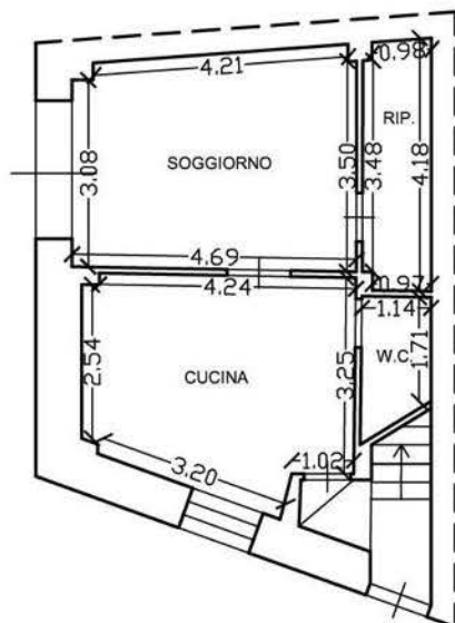
PIANTA PIANO TERRA - h = m 2.65
