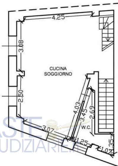
PIANTA PIANO PRIMO - h = m 2.73
