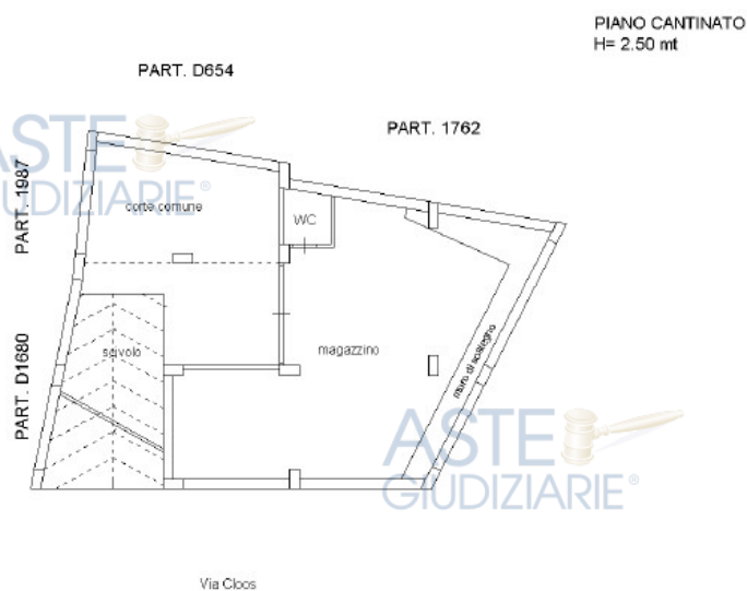
FIGURA 15 – PLANIMETRIA CATASTALE
