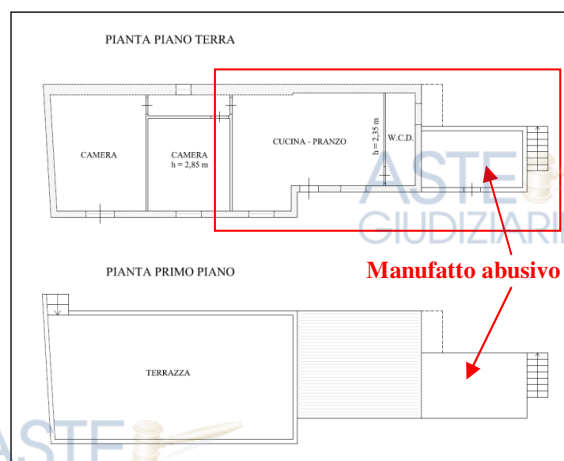
Rilievo stato attuale dei luoghi)
