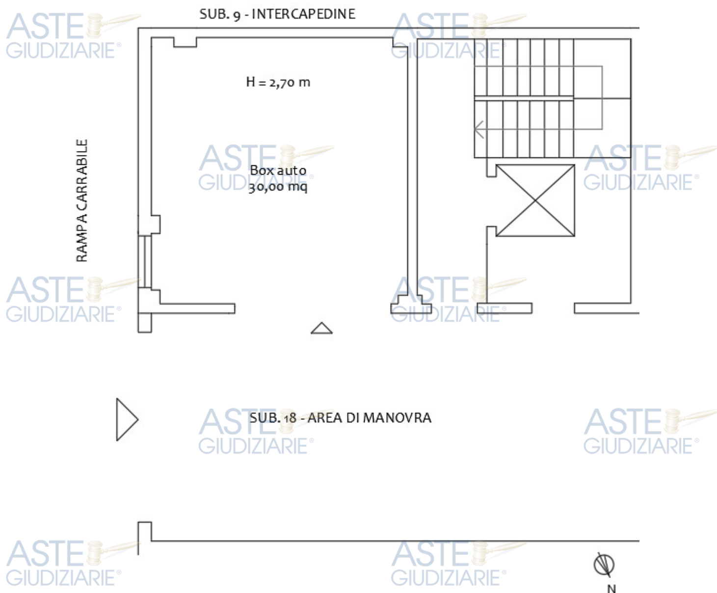
Figura 4: Planimetria box auto
