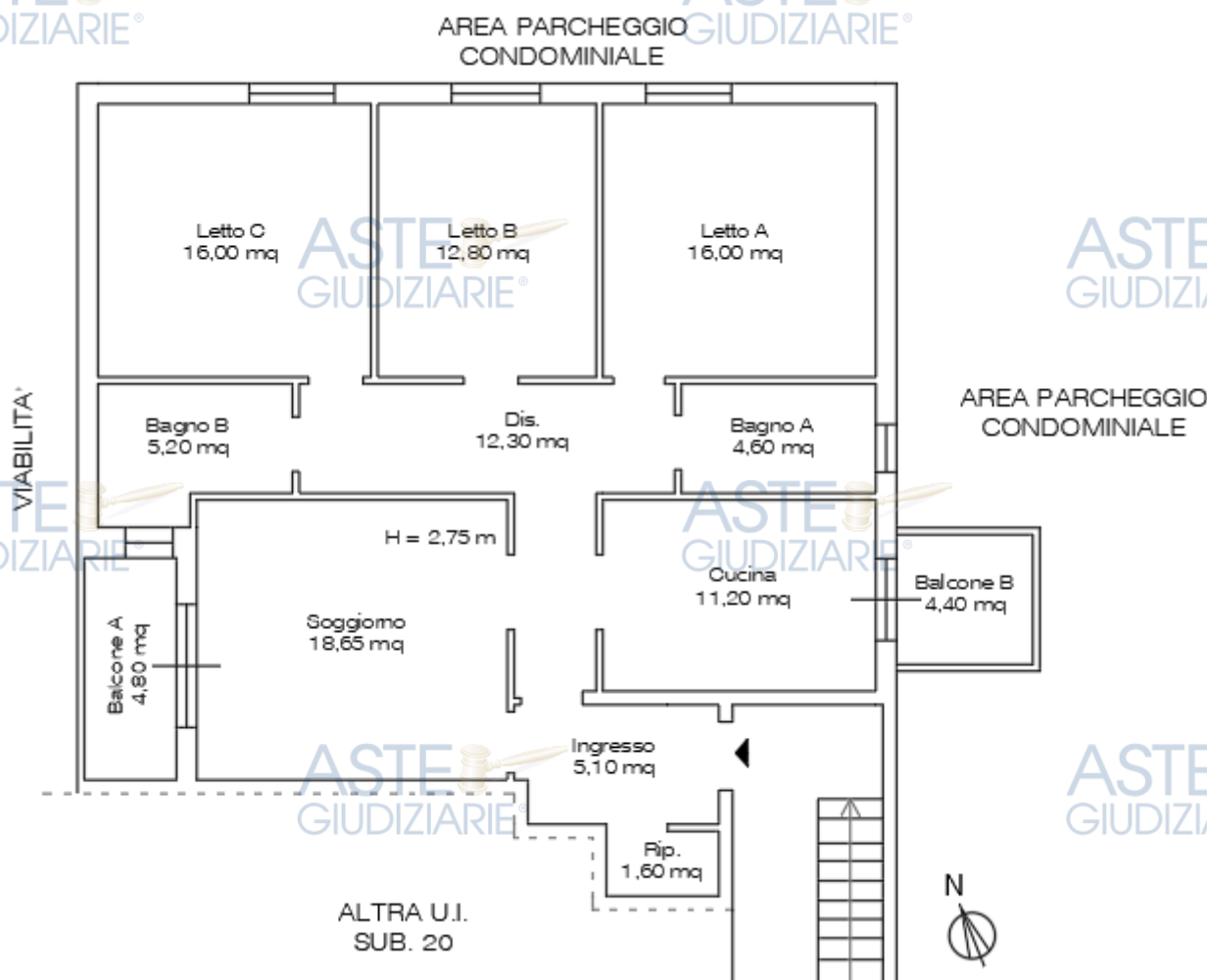
Figura 4: Planimetria immobile
