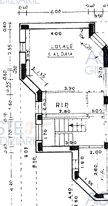
Pianta piano seminterrato da Concessione Edilizia
