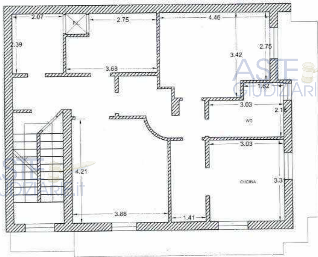
piano piano secondo _ scala 1:100
