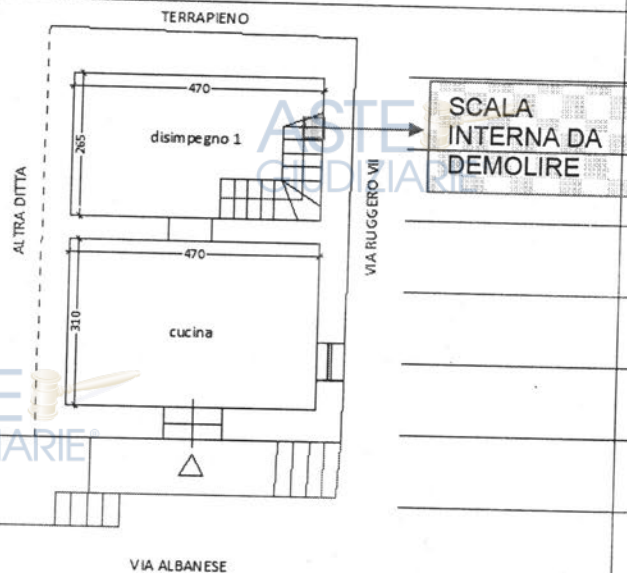
Figura 1. LOTTA B - Pianta piano terra STATO DI FATTO
