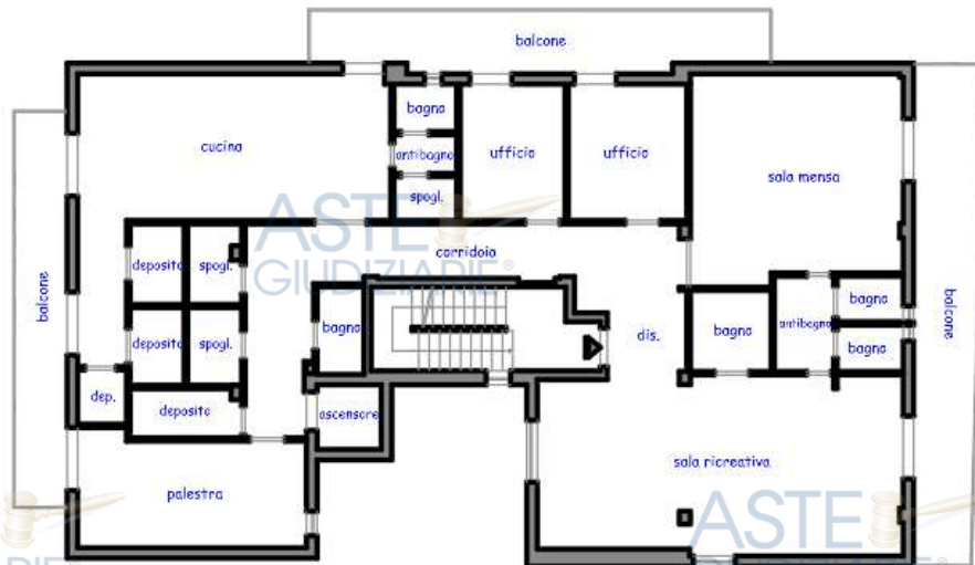
Planimetria dello stato di fatto - Piano Primo
