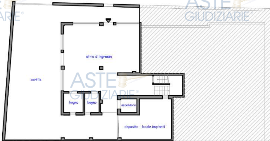
Planimetria dello stato di fatto - Piano Terra
