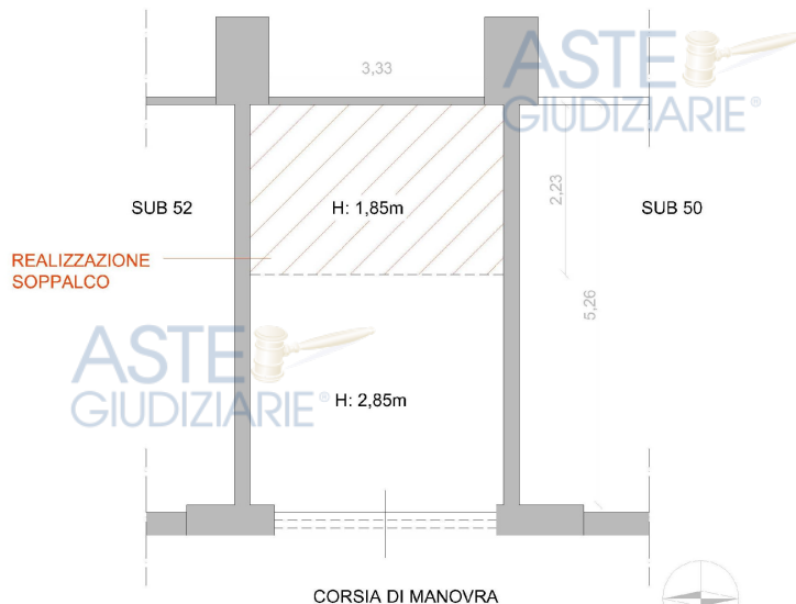
GRAFICI DI RILIEVO CON INDICAZIONE DELLE DIFFORMITA' CATASTALI - BOX AUTO SITO AL PIANO S1, SCALA B, - CASAPULLA (CE) VIA A. DIAZ, N. 48 - IN CATASTO AL FOGLIO 5, P.LLA 5001, SUB 51, CAT. C/6. - SCALA 1:100
