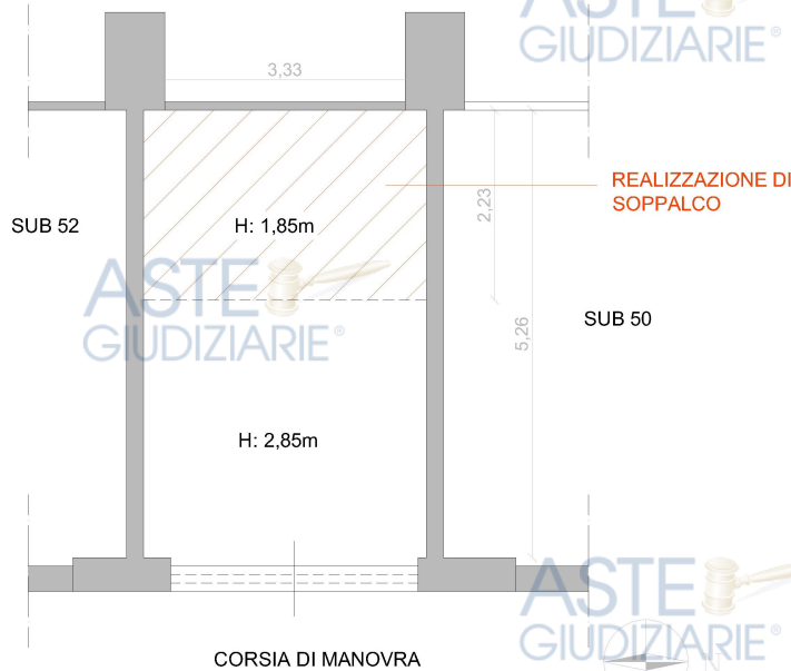
GRAFICI DI RILIEVO CON INDICAZIONE DELLE DIFFORMITA' EDILIZIE - BOX AUTO SITO AL PIANO S1, SCALA B, - CASAPULLA (CE) VIA A. DIAZ. N. 48 - IN CATASTO AL FOGLIO 5, P.LLA 5001, SUB 51, CAT. C/6. - SCALA 1:100
