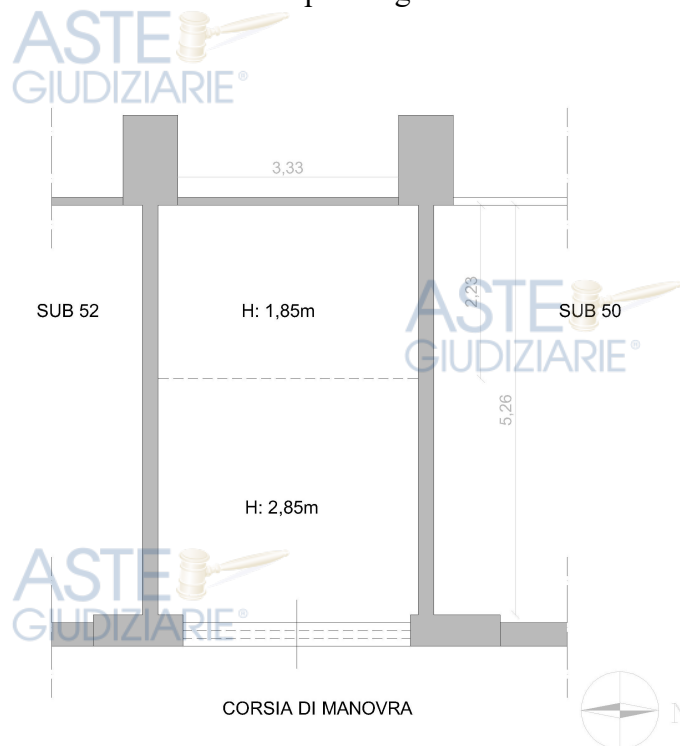
GRAFICI DI RILIEVO - BOX AUTO SITO AL PIANO S1, SCALA B, - CASAPULLA (CE) VIA A. DIAZ, N. 48 - IN CATASTO AL FOGLIO 5, P.LLA 5001, SUB 51, CAT. C/6. - SCALA 1:100
