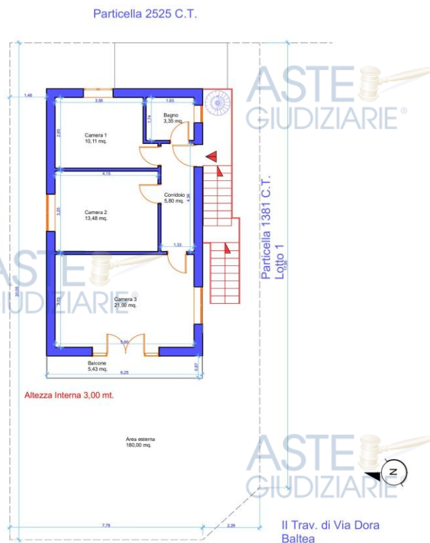
Piano primo (sub 2)
