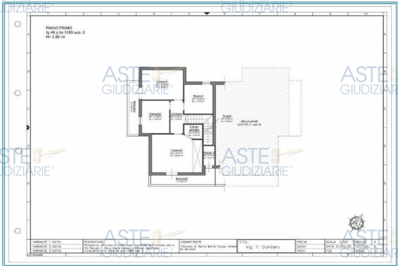
Figura 13 Stato attuale - Piano Primo (LOTTO 1)
