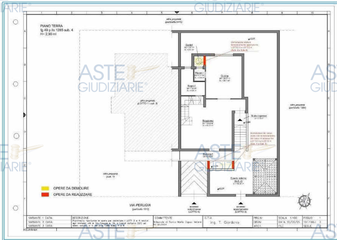
Figura 9 Rappresentazione delle opere necessarie alla separazione dei LOTTI 3 e 4 - (Piano Terra - LOTTO 3)
