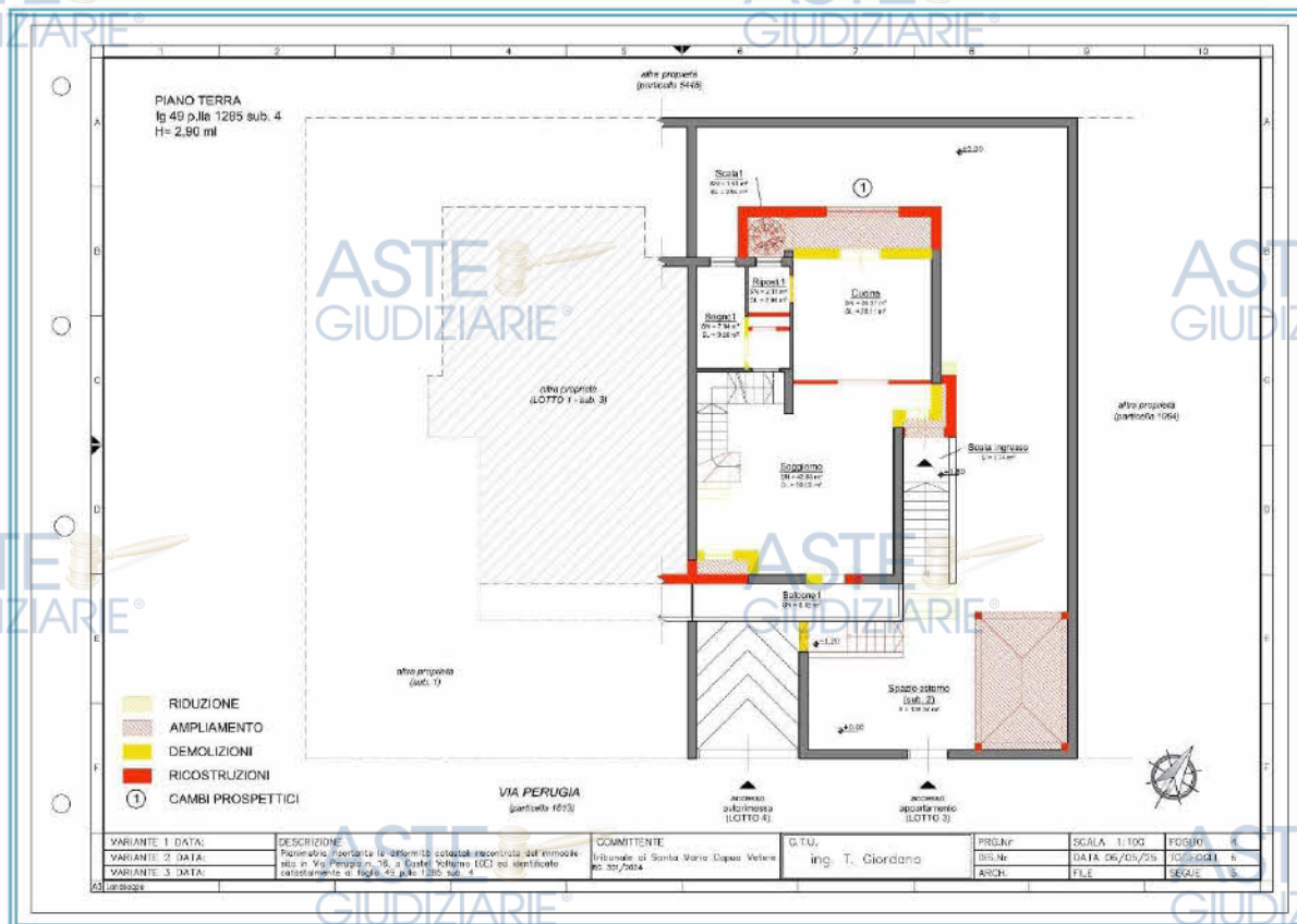
Figura 82 Schema diffinitività catastali - Piano Terra (LOTTO 3)
