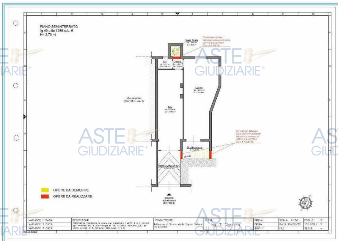
Figura 10 Rappresentazione delle opere necessarie alla separazione dei LOTTI 3 e 4 - (Piano Seminterrato - LOTTO 4)
