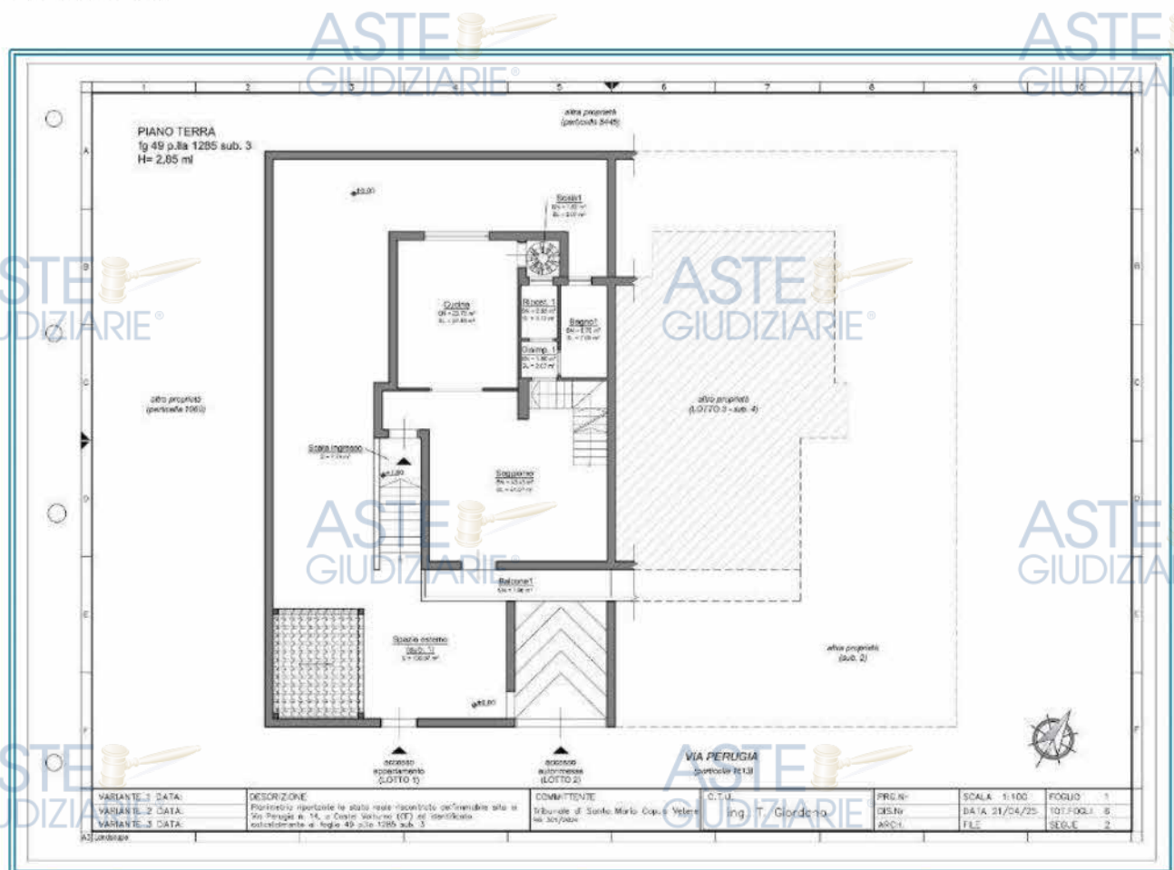
Figura 12 Stato attuale - Piano Terra (LOTTO 1)
