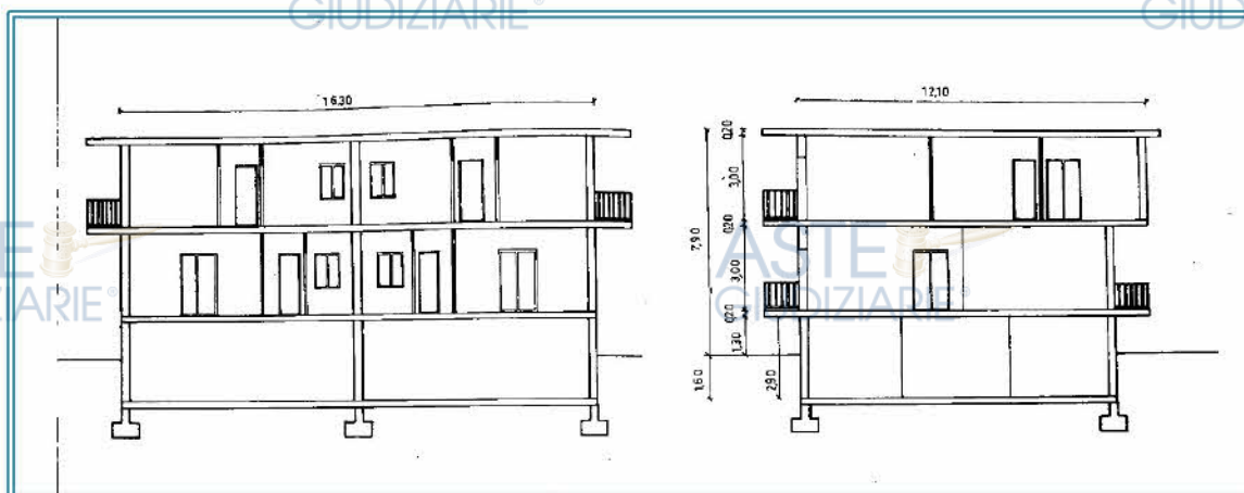
Figura 92 Sezioni – estratto dal fascicolo pratica di condono n. 8104/86
