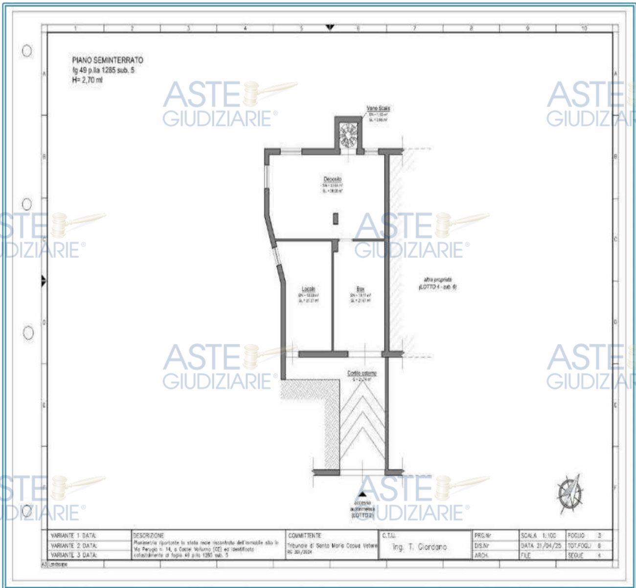
Figura 32 Stato attuale - Piano Seminterrato (LOTTO 2)
