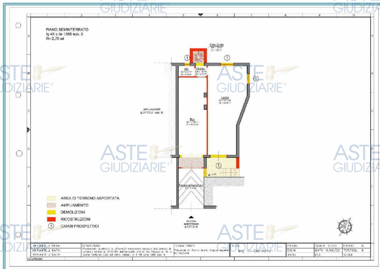
Figura 99 Schema difformità urbanistiche piano seminterrato (LOTTO 4)
