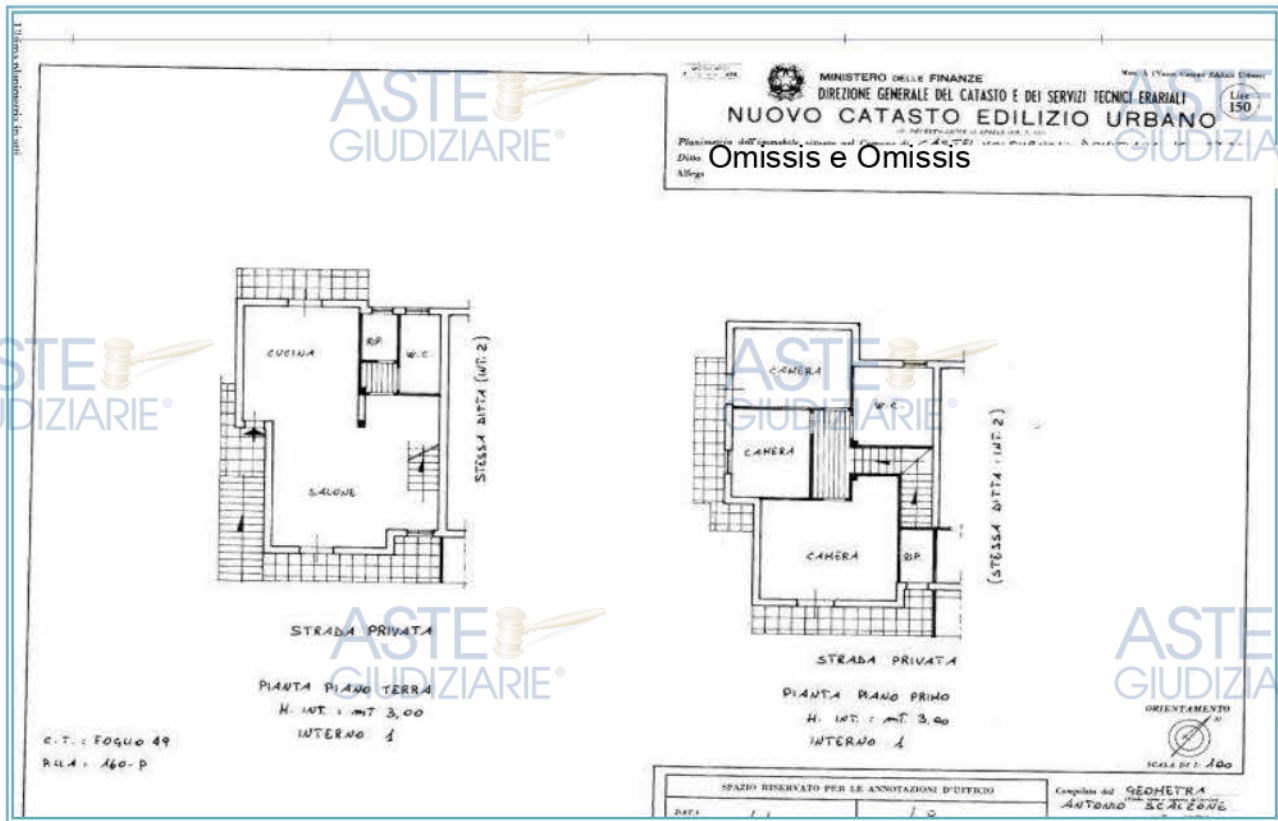
Figura 76 Pianta catastale attuale – Piano Terra e Primo (LOTTO 1)
