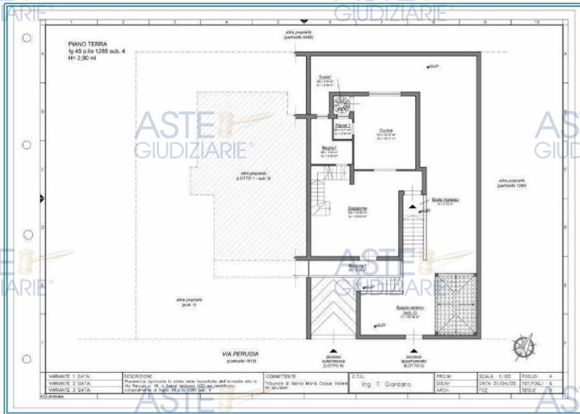
Figura 39 Stato attuale - Piano Terra (LOTTO 3)
