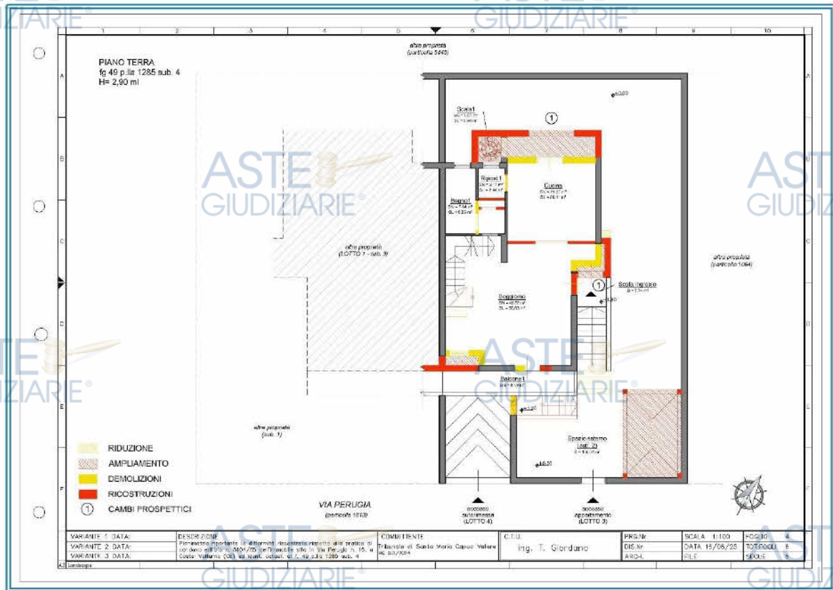
Figura 97 Schema difformità urbanistiche piano terra (LOTTO 3)
