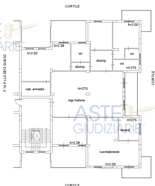
Figura 41 planimetria catastale dell'appartamento mansardato al quinto piano
