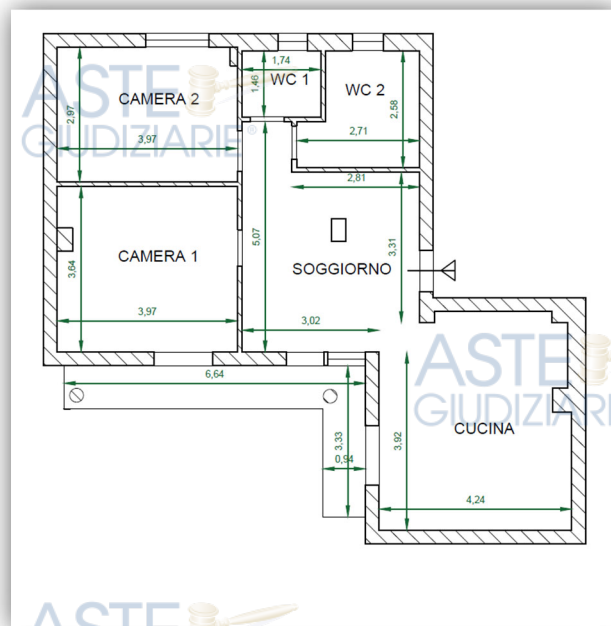
Fig. 500 P.lla 2072 Sub 17 – stato attuale al ...OMISSIS...
