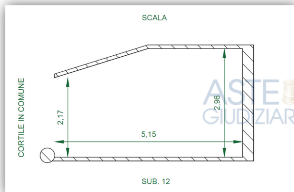
Fig. 500 P.lla 2072 Sub 13 – stato attuale al ...OMISSIS...
