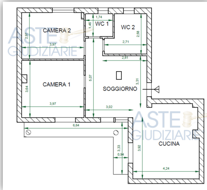
Sub 17 – Stato attuale al ...OMISSIS...
