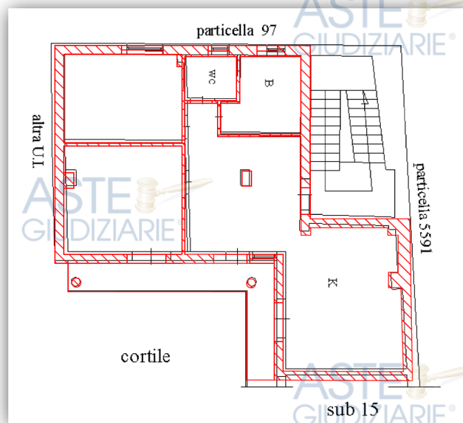
Sovrapposizione planimetria catastale – planimetria di rilievo relativamente al Sub .17
