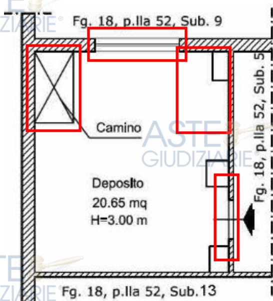
Pianta immobile staggito (sub 7 piano terra) - Rilievo esperto
