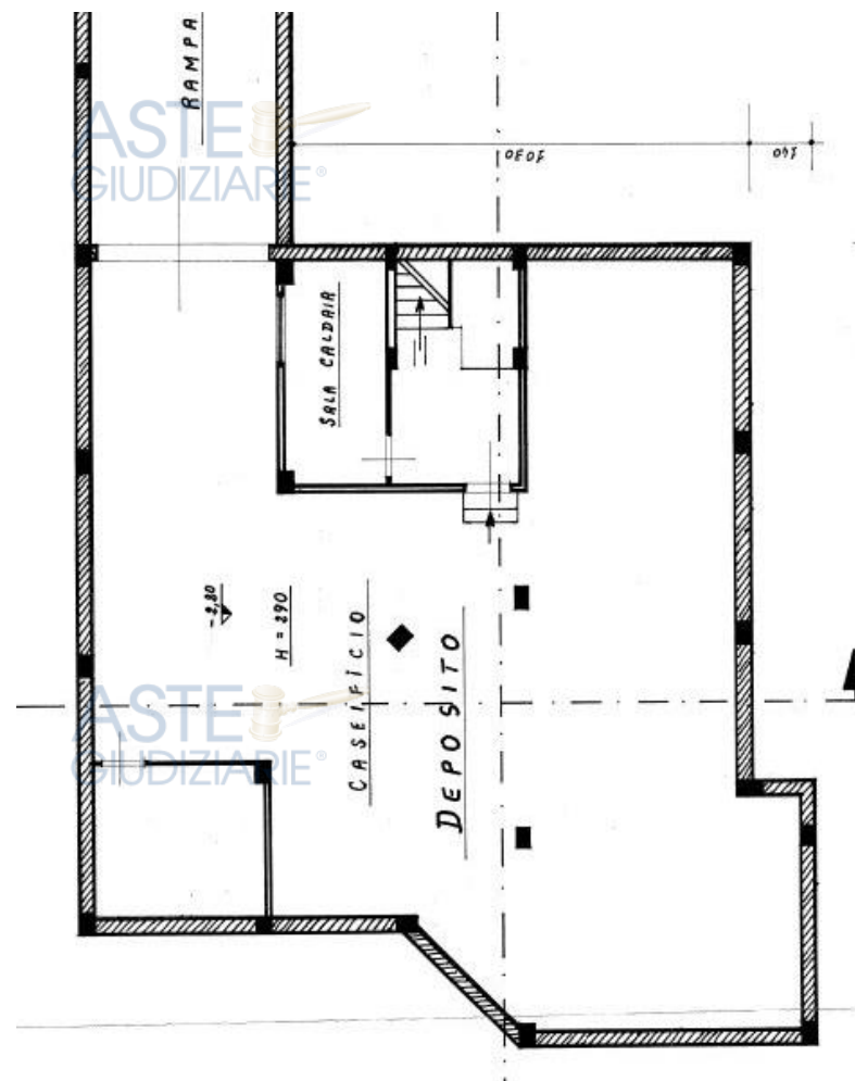
Pianta sub 7 interrato – C. E. in Sanatoria n. 30/2003 del 17/11/2003
