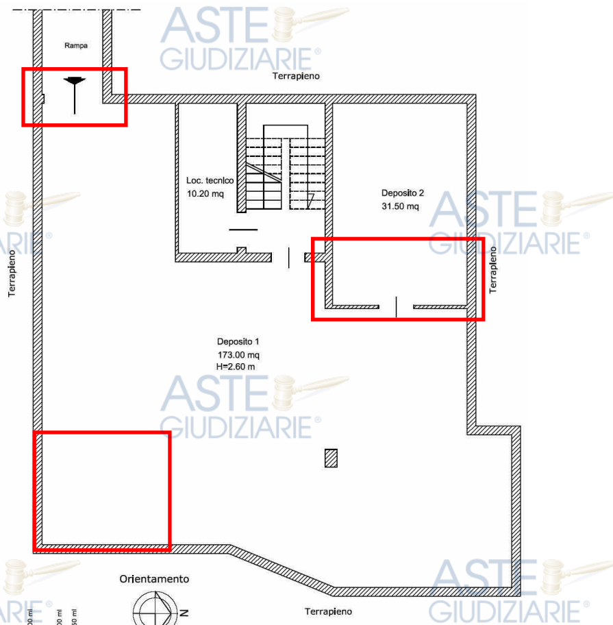
Pianta immobile staggito (sub 7 piano interrato) - Rilievo esperto
