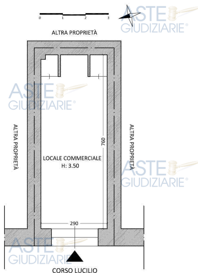
Rilievo stato dei luoghi
