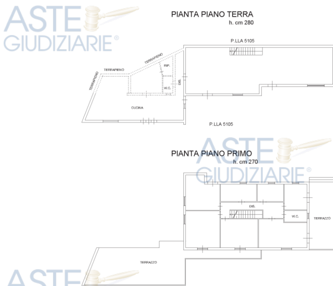
Figura 80 planimetria catastale del piano terra e del primo piano della villa – sub 3
