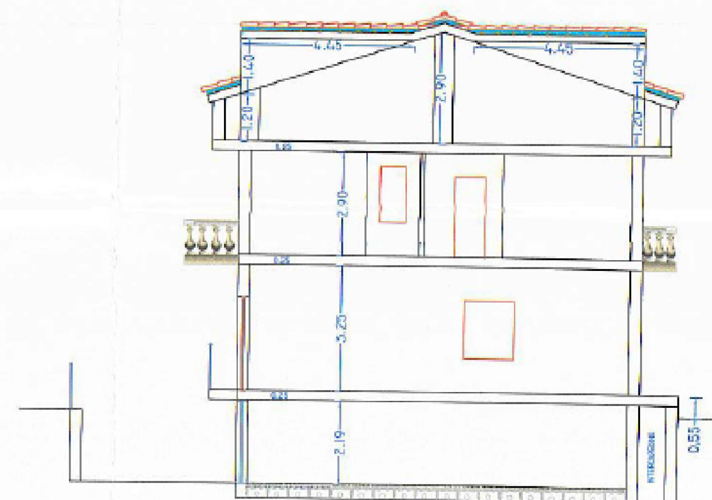
SEZIONE B - B
