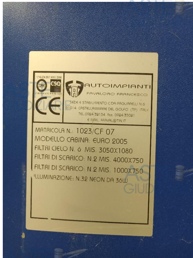
Foto n. 33 - CABINA VERNICIATURA
