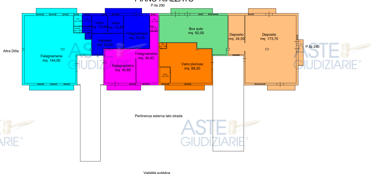
Fig. 5: Rilievo generale del piano rialzato ed individuazione delle 3 unità immobiliari per ogni corpo di fabbrica
