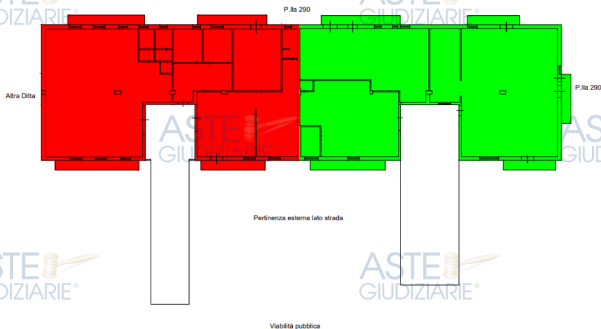
Fig. 1: Rilievo generale degli immobili ed individuazione dei due corpi di fabbrica
