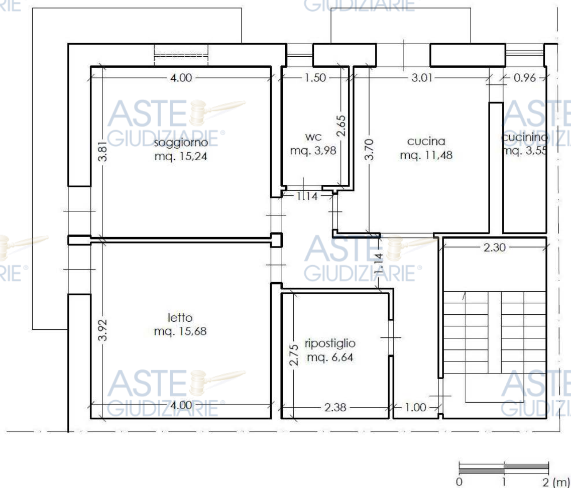
PLANIMETRIA IMMOBILE STATO ATTUALE
