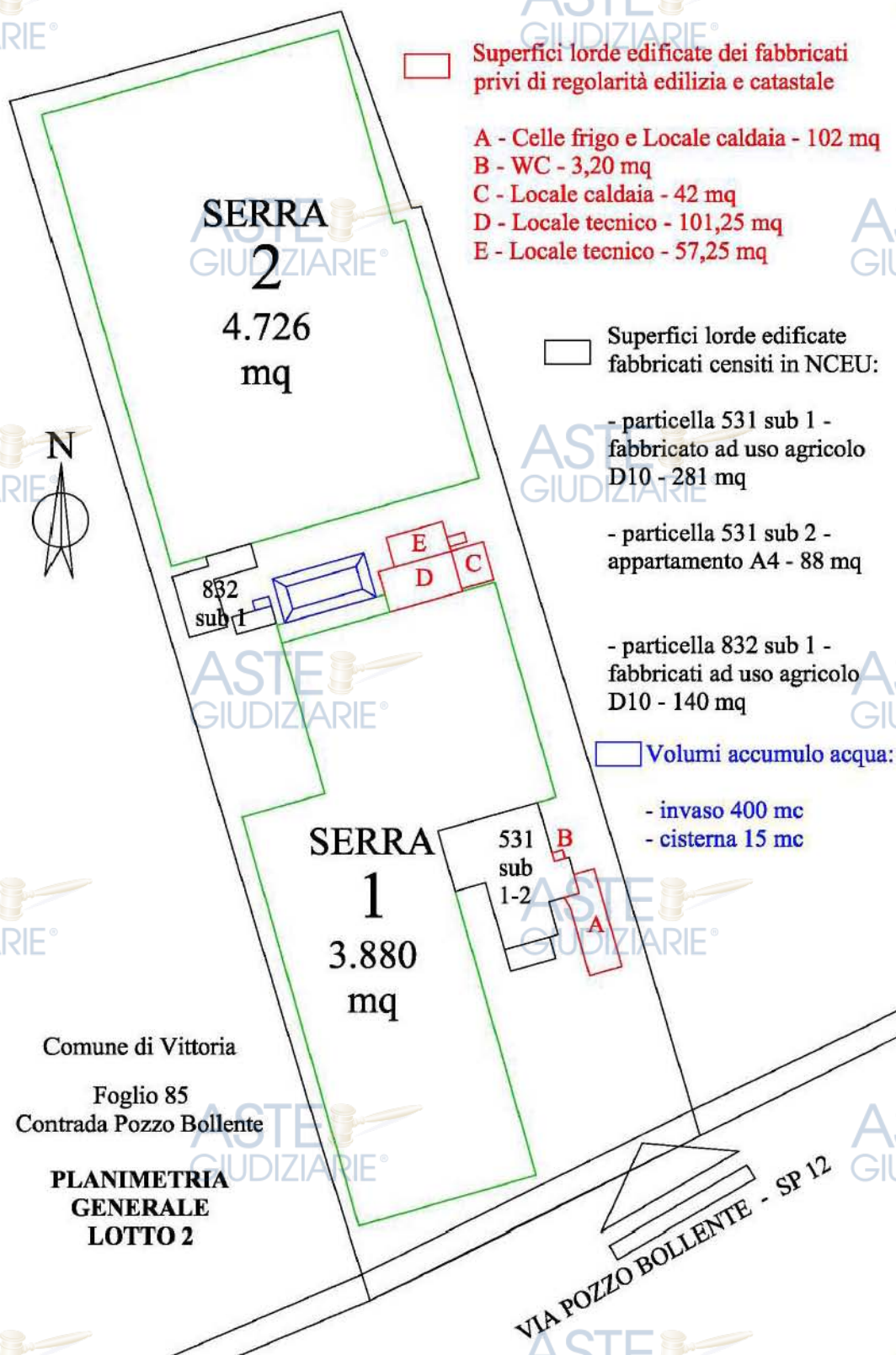
Figura 11 – Lotto 2 – Planimetria generale
