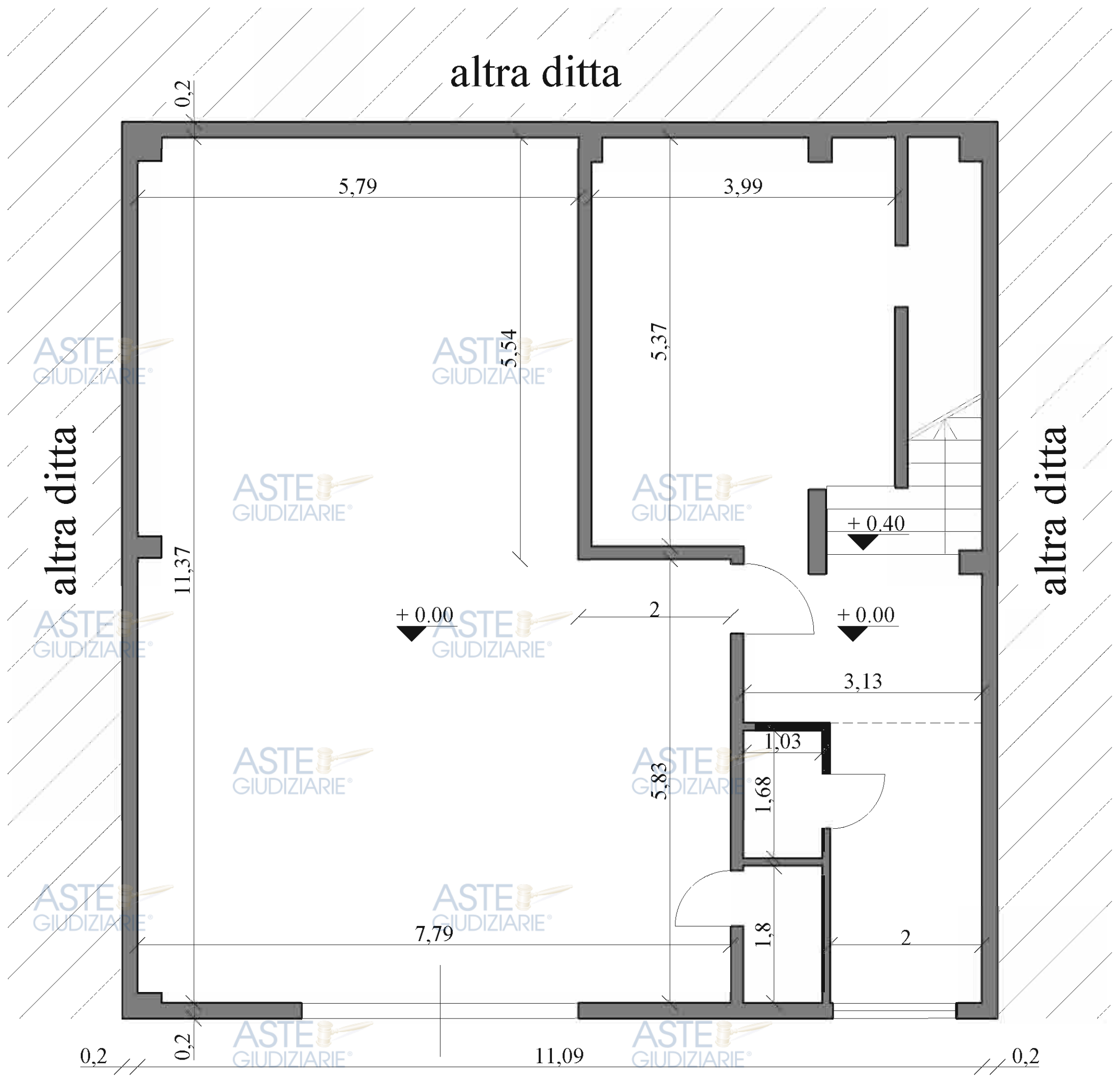
via Manzoni pianta piano terra
