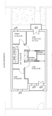
PLANIMETRIA PIANO Primo sub 7
