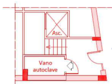
Figura 8 - Sovrapposizione planimetria dello stato reale dei luoghi con la planimetria catastale - Vano autoclave Piano Terra
