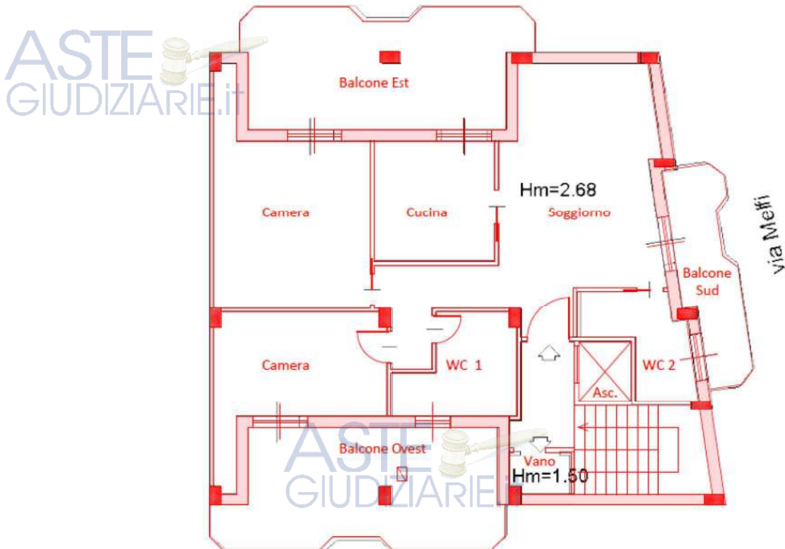
Figura 9 – Sovrapposizione planimetria dello stato reale dei luoghi con la planimetria catastale - Appartamento Piano Quarto
