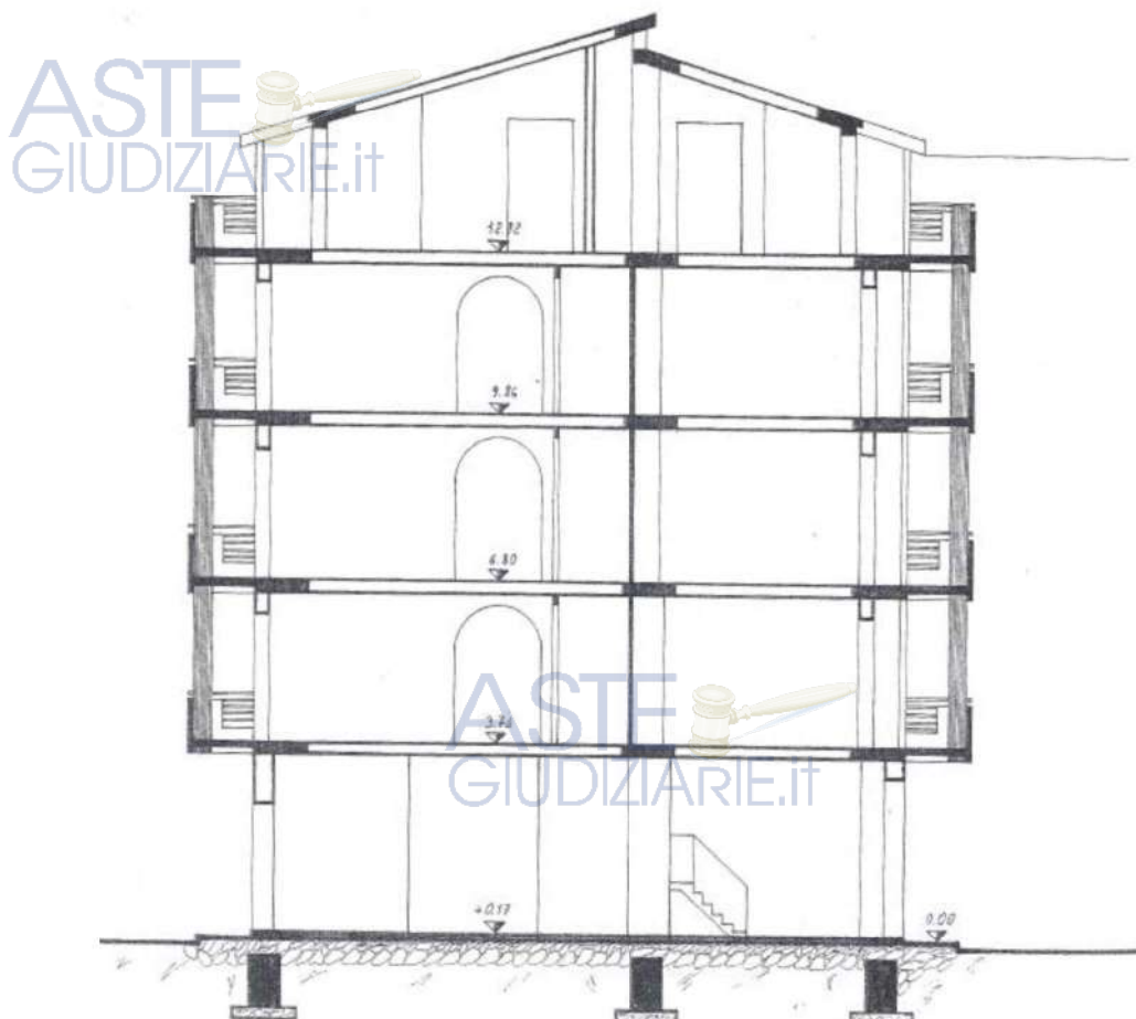
Figura 11 - Sezione trasversale Conc. Ed. n. 33/1995
