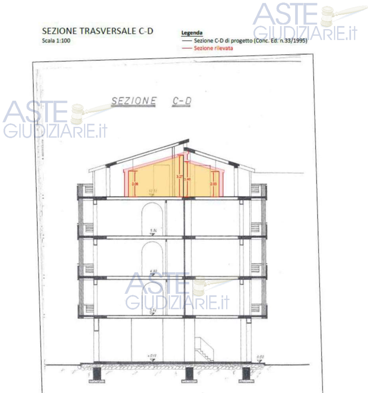
Figura 13 - Sovrapposizione stato reale dei luoghi e progetto autorizzato – Sezione trasversale C-D
