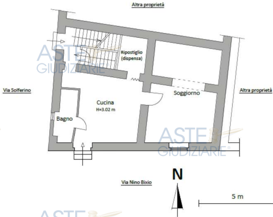
Figura 6 - Planimetria dello stato reale dei luoghi - Piano Terra
