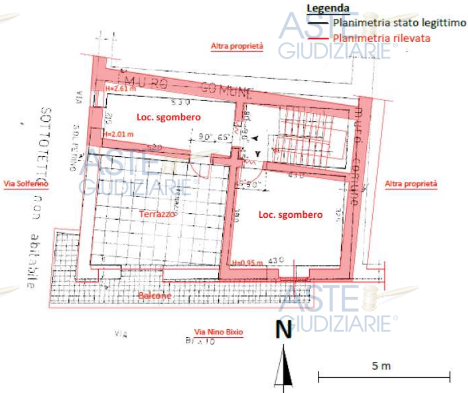
Figura 18 - Sovrapposizione stato reale dei luoghi e progetto autorizzato - Planimetria Piano 2°
