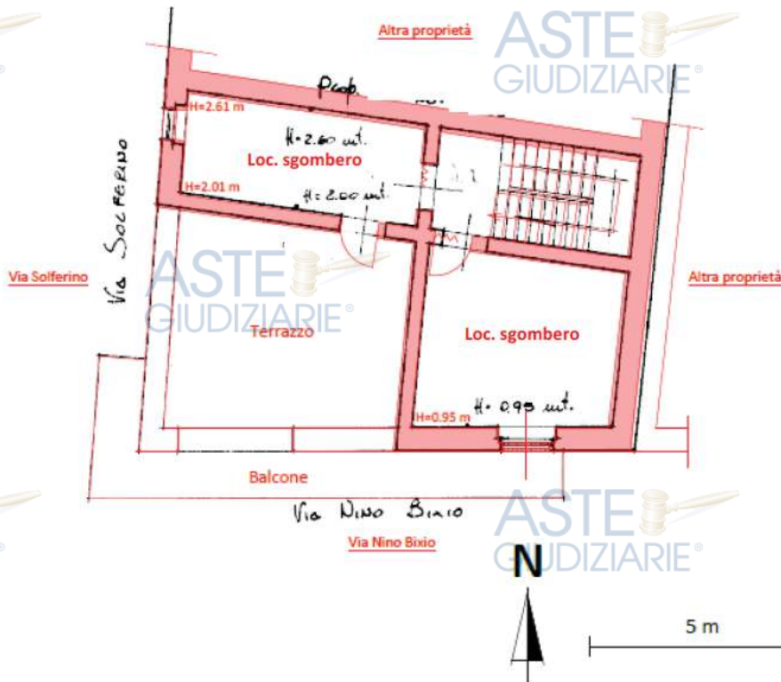
Figura 12 - Sovrapposizione planimetria dello stato reale dei luoghi con la planimetria catastale - Piano 2°
