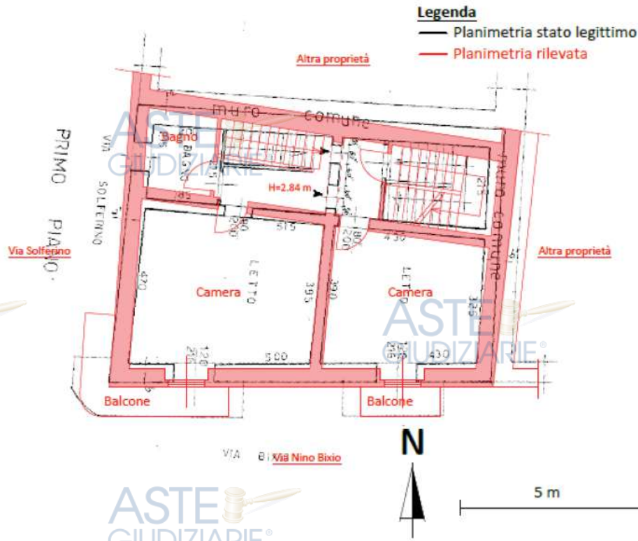
Figura 17 - Sovrapposizione stato reale dei luoghi e progetto autorizzato - Planimetria Piano 1°
