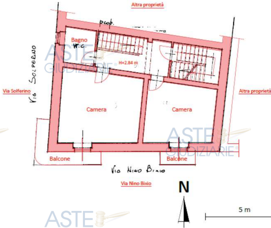
Figura 11 - Sovrapposizione planimetria dello stato reale dei luoghi con la planimetria catastale - Piano 1°
