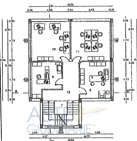
foglio 8 part. 256 PIANO TERRA
